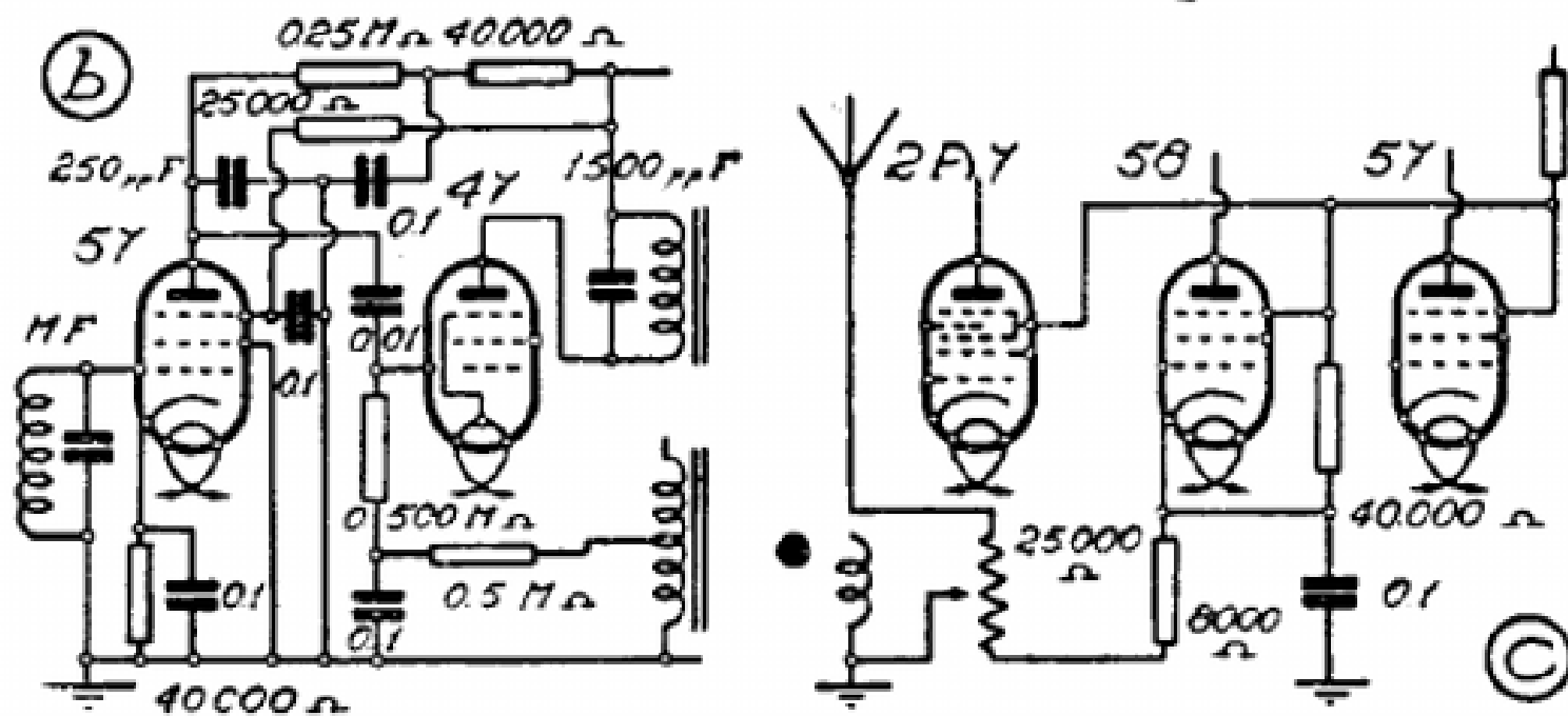
Varianti per i modelli Watt in (a) il « 659 », in (b) e (c) il mod. « Ardito ».
